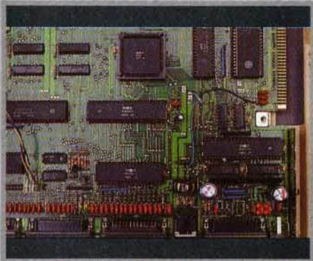
La carte de l'Amiga 500, petit frère de l'Amiga 1000 et père de l'Amiga 300+ et 600. Très controversée à sa sortie, cette superbe machine a fini par ... plaire.
